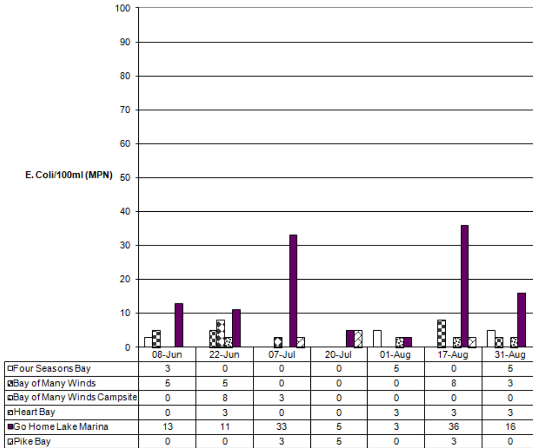
Go Home Lake E. Coli 2019
